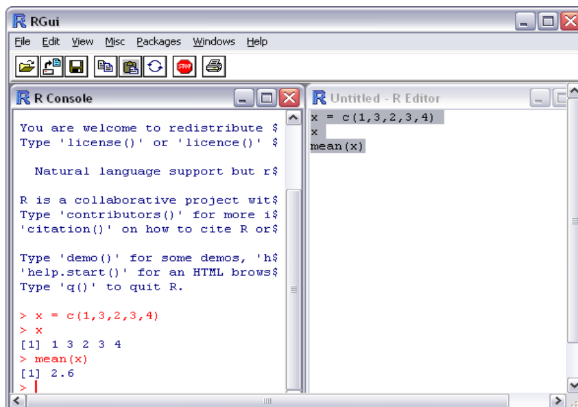
Figura 1.2. Console do programa R ilustrando a janela de script , em que um programa é executado e apresenta a definição de um vetor, sua impressão e o cálculo da média.
