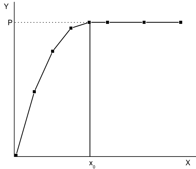
Figura 4.2. Modelo segmentado considerando um plateau no ponto X = X_0 com valor de Y = P e um modelo crescente para X < X_0 .
