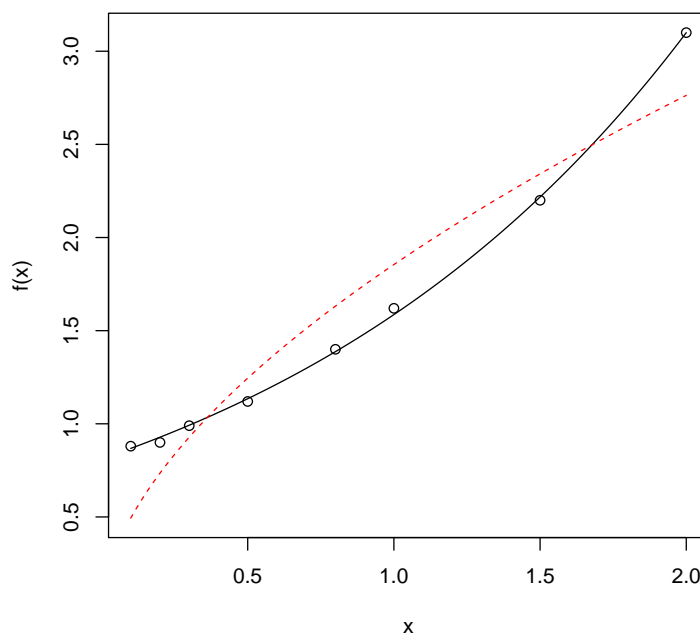
Figura 4.1. Modelos não lineares ajustados - modelo \hat{y}_i = 1,8548x_i^{0,575} em vermelho e modelo \hat{y}_i = 0,8117 \times 1,9542^{x_i} em preto.
