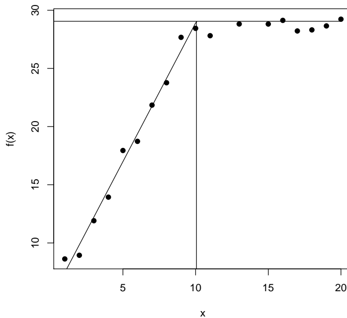
Figura 4.5. Modelo platô de resposta linear ajustado: \hat{Y}_i = 5,0731 + 2,3834X_i se X_i \leq 10,06 e \hat{Y}_i = 29,05 , se X_i > 10,06 .
