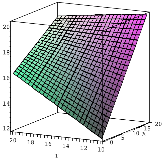
Figura 5.1. Modelo ajustado de superfície de resposta para os dados de produção em função da adubação mineral ( AM ) e da adubação orgânica com torta de filtro ( TF ).
