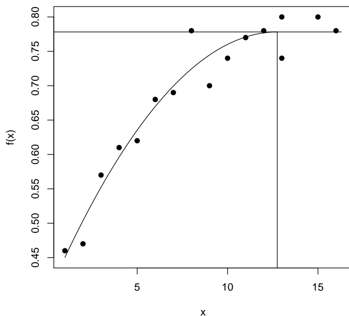
Figura 4.3. Modelo platô de resposta ajustado \hat{Y}_i = 0,3921 + 0,0605X_i - 0,00237X_i^2 se X_i < 12,7477 e \hat{Y}_i = 0,7775 , caso contrário.
