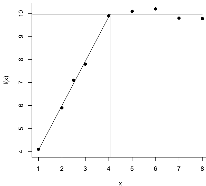
Figura 4.4. Modelo platô de resposta linear ajustado: \hat{Y}_i = 2,135 + 1,93X_i se X_i \leq 4,06 e \hat{Y}_i = 9,97 se X_i > 4,06 .
