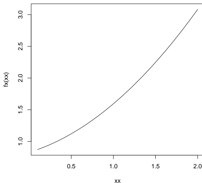
Figura 3.1. Equação quadrática resultante do ajuste de quadrados mínimos do exemplo.
